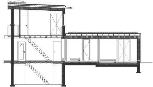
Schnitt A
